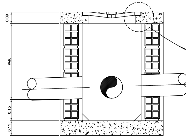
CORTE AA'
