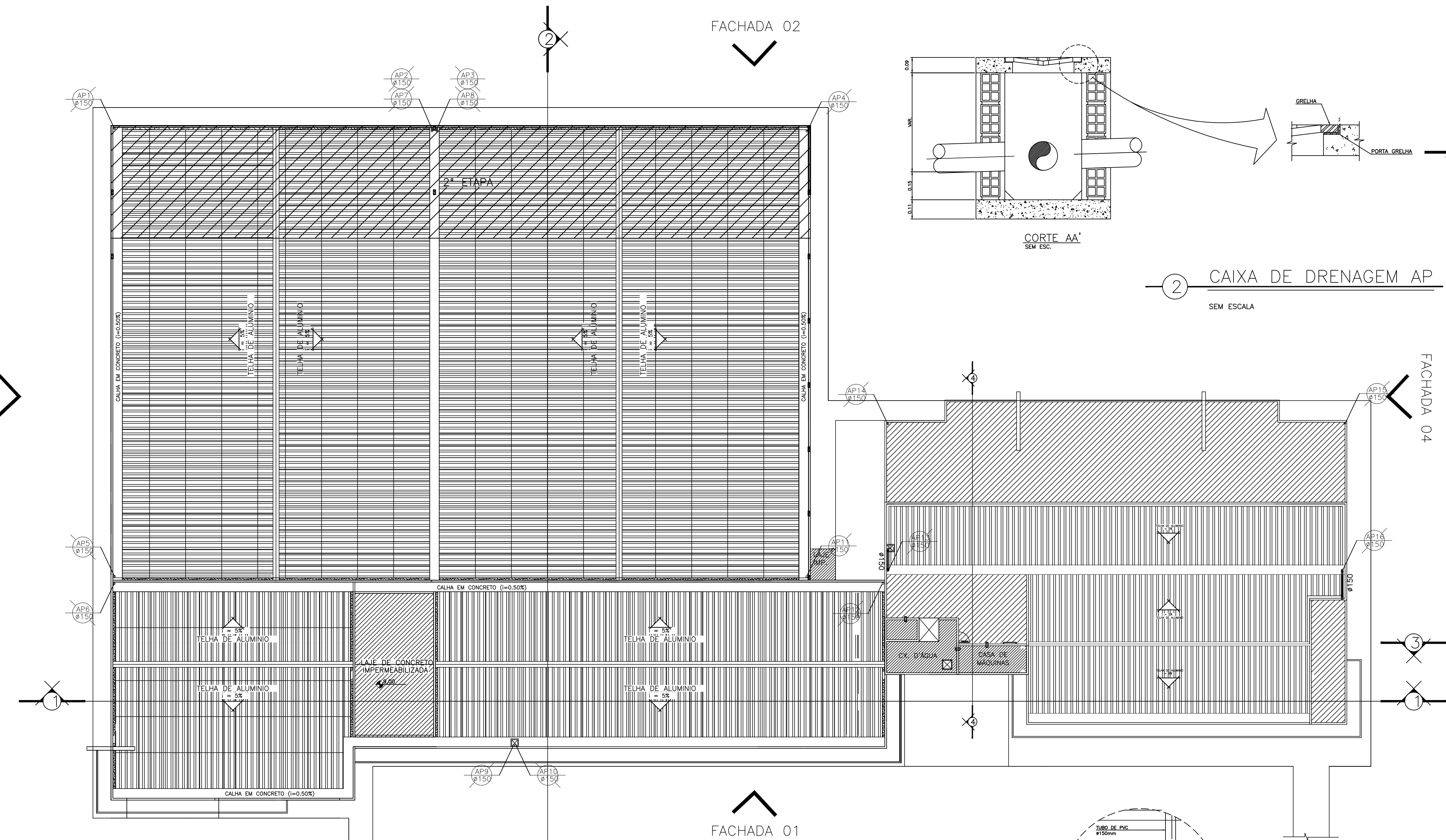
1 PLANTA BAIXA DE COBERTURA
