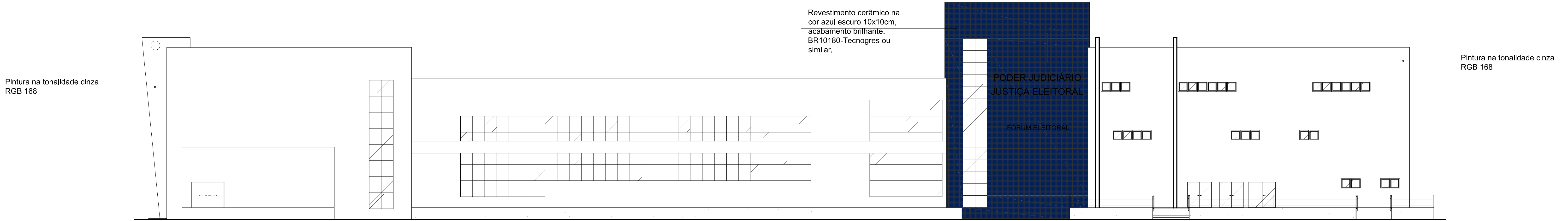
FACHADA 02 ESC.: 1/150
