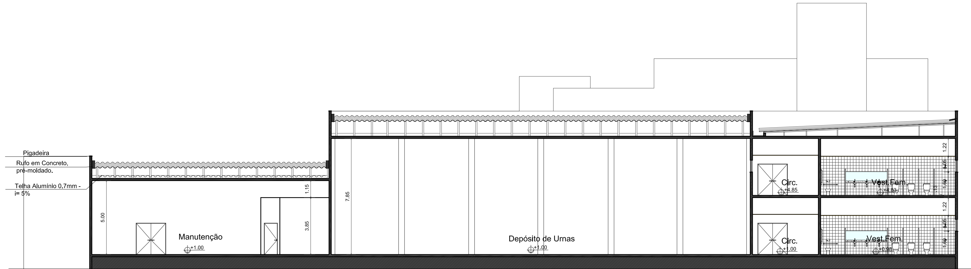
CORTE 02 ESC: 1/150
