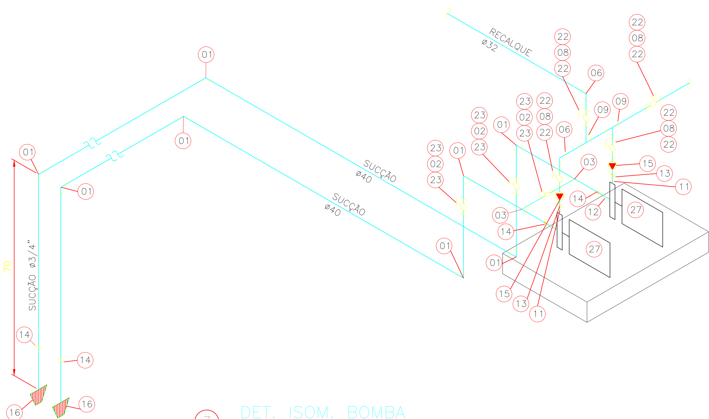
3 DET. ISOM. BOMBA SEM ESCALA
