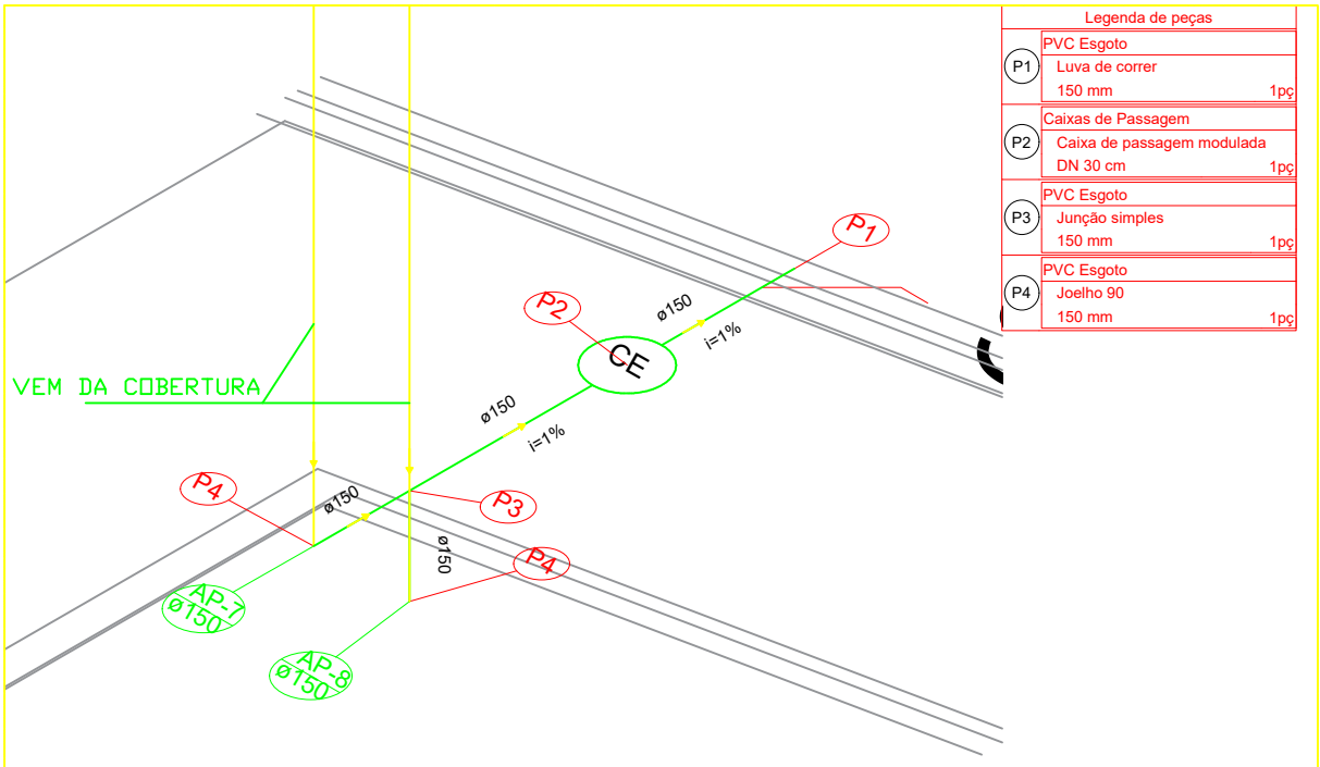
DETALHE ISOMÉTRICO-S10 SEM ESCALA
