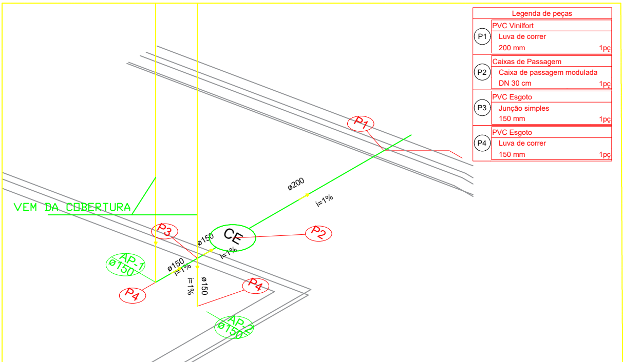
DETALHE ISOMÉTRICO-S09 SEM ESCALA
