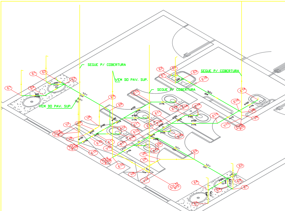
DETALHE ISOMÉTRICO-S12 SEM ESCALA
