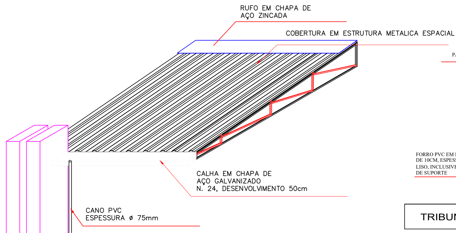
2 PERSPECTIVA 1
