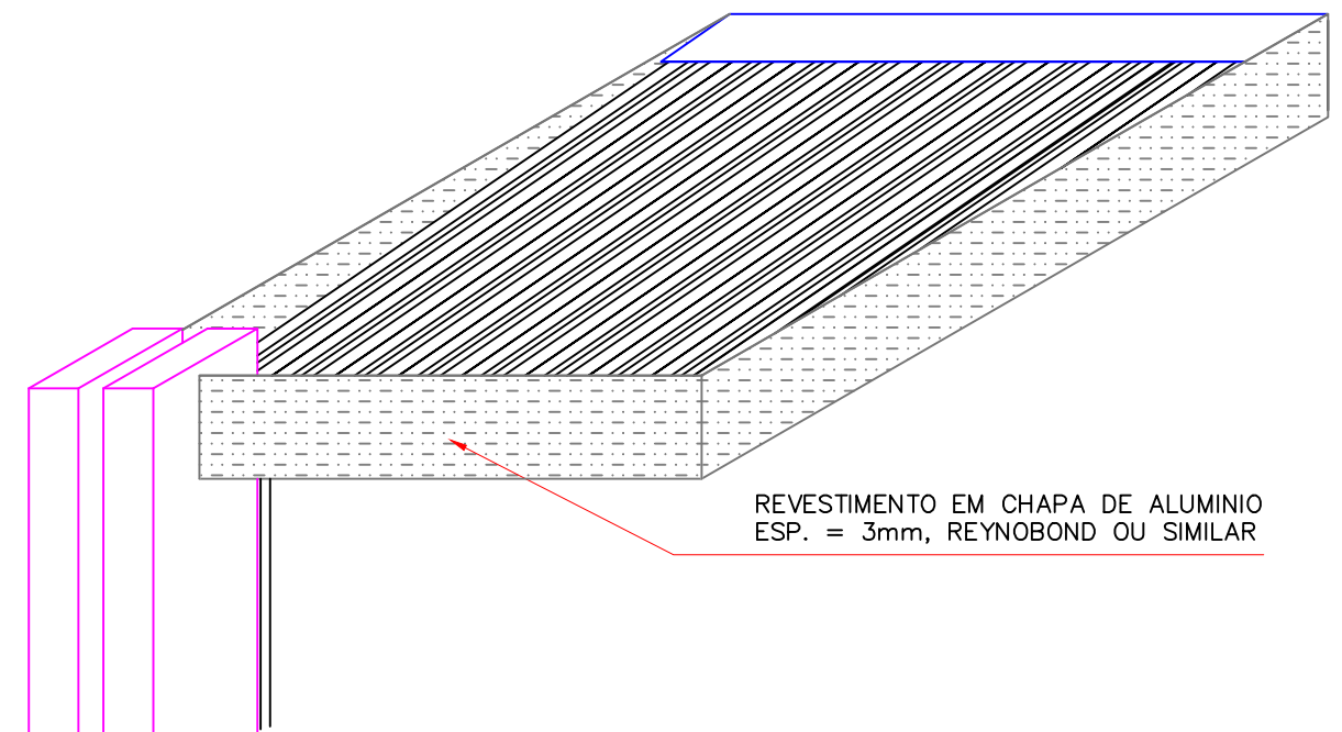
2 PERSPECTIVA 2
