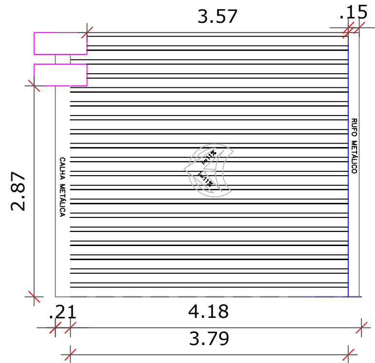
1 PLANTA DE COBERTURA DA MARQUISE
