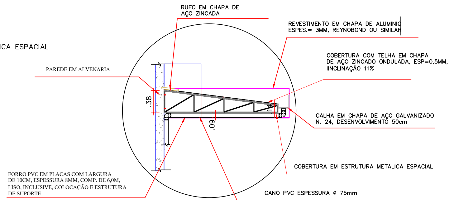
4 VISTA LATERAL
